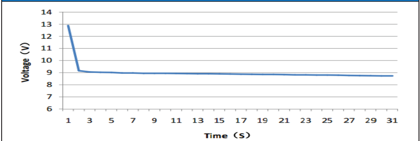
Cold Cranking Test Graph (-18°C, 1000CCA)
